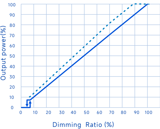
输出功率Vs.调光信号
